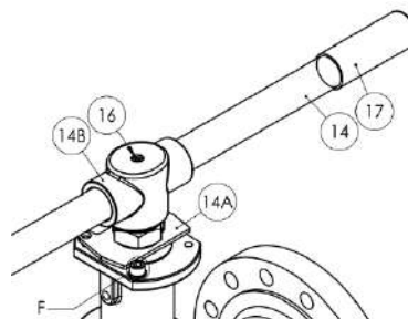
Detalle B:
