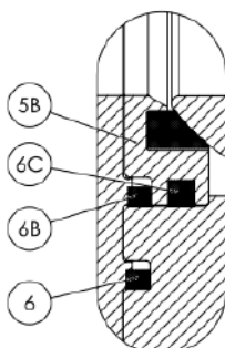
Detalle B-2
