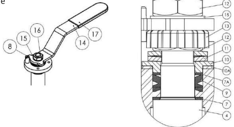
Detalle A:
